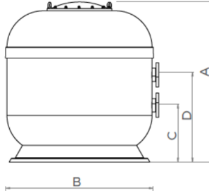
Dimensions d950-1400
