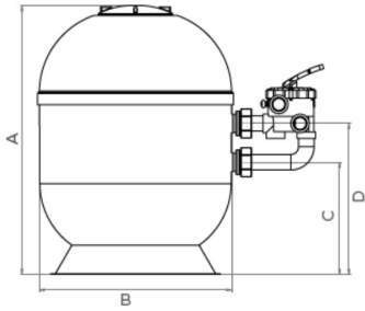
Abmessungen d400 - d900
