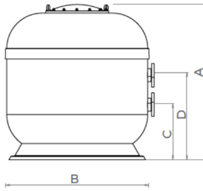
Abmessungen d950-1400
